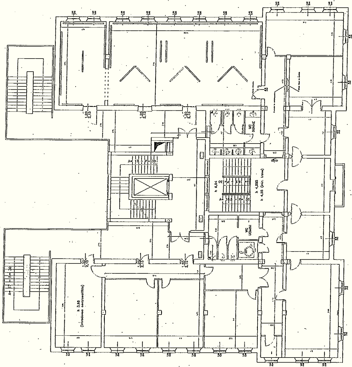
PIANTA LIVELLO 3 (PIANO PRIMO)
